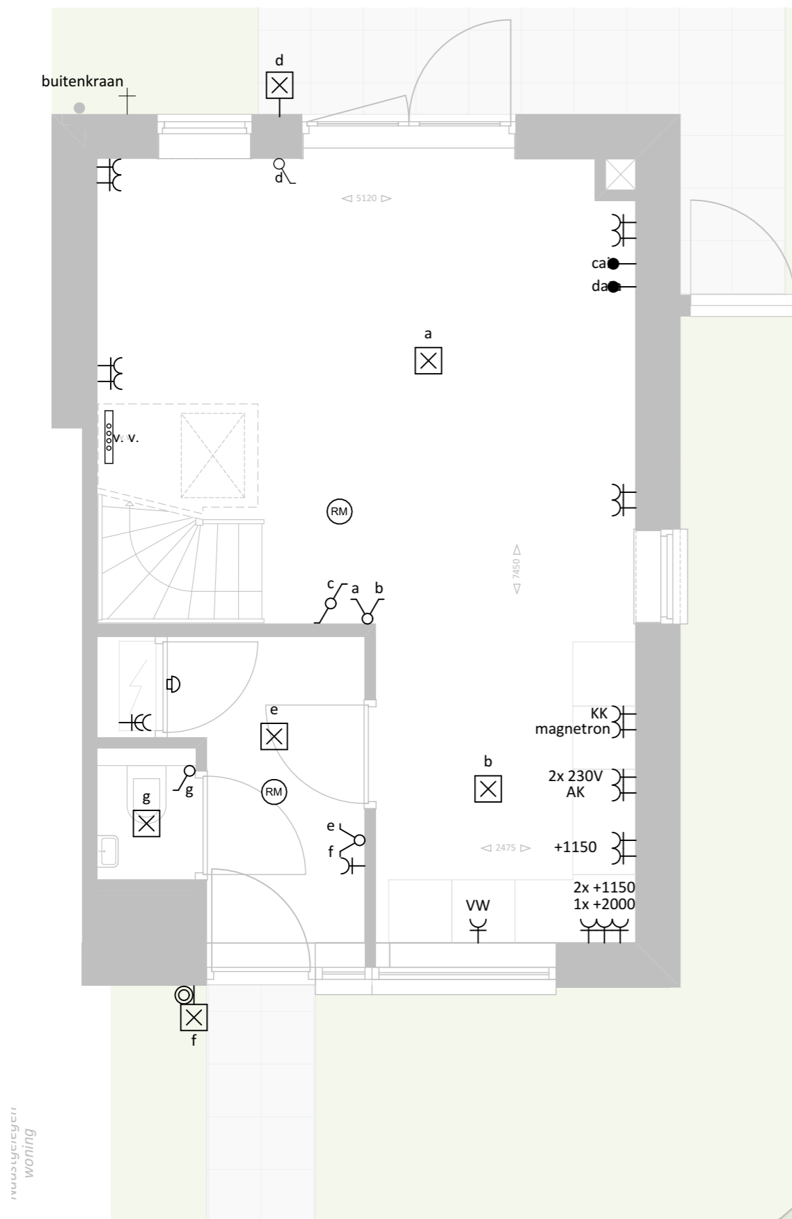
Begane grond
